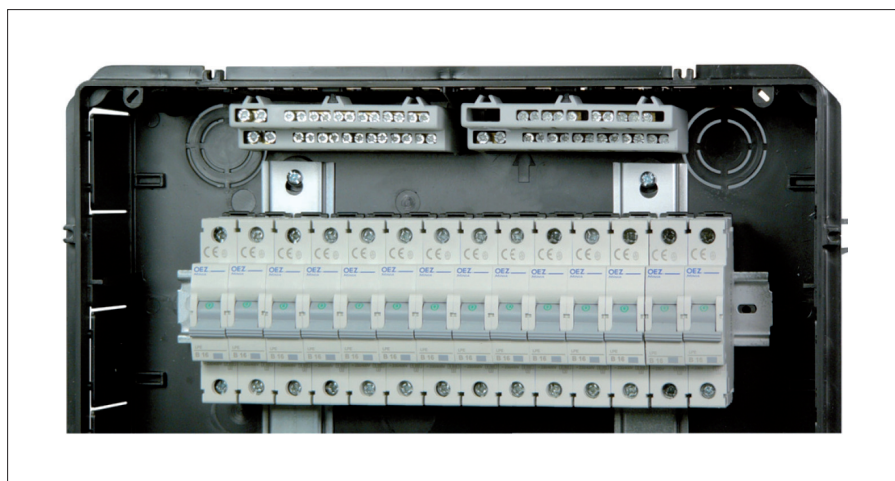
Obr. 5. Dostatečný prostor pro vodiče
