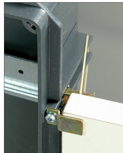
Obr. 6. Upevnění do sádrokartonových příček
